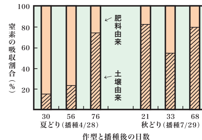
レタスの吸収窒素の由来別割合
