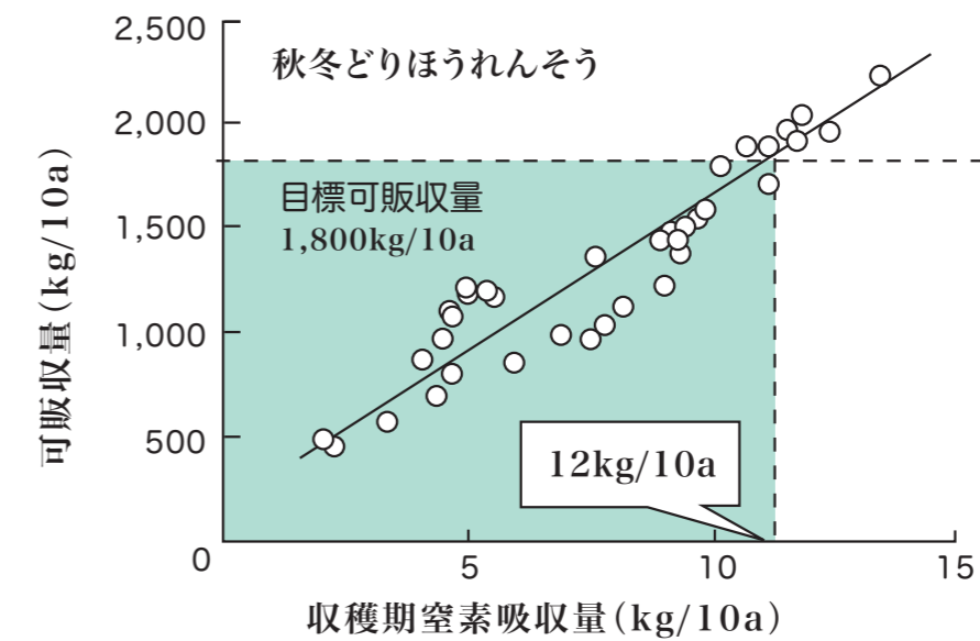
秋冬どりほうれんそうの窒素吸収量と可販収量との関係 (資料：千葉県農試)
